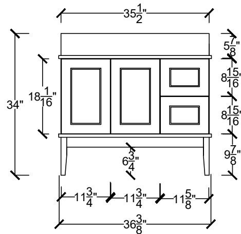
RANV 3622 2DL OR 2DR-____-____-
