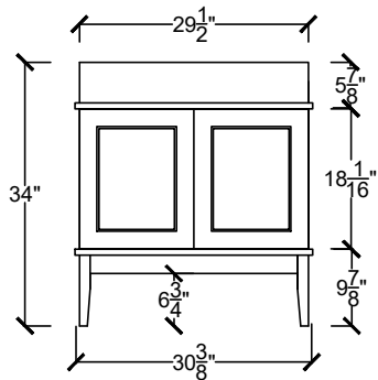
RANV 3022- - - RANV 3019- - -
