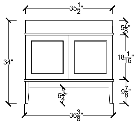
RANV 3622-____-____-
