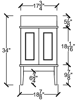
RANV 1917- - -
